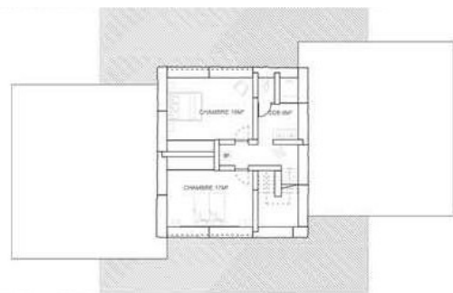
Détail RDC d'un lodge 4 personnes
