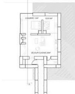
Détail RDC d'un lodge 2 personnes
